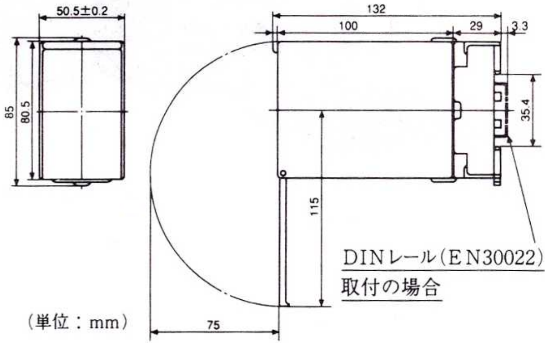
FAL -100 -1外形寸法図
