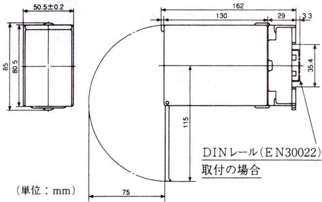
FAL-100-3外形寸法図
