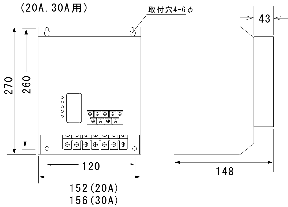
FPG-3外形寸法图
